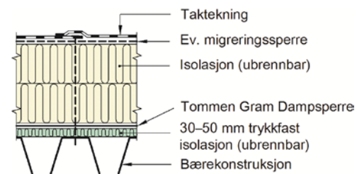
Fig. 1 Tommen Gram Dampsperre og Tommen Gram Grønn Dampsperre montert i massiv takkonstruksjon
